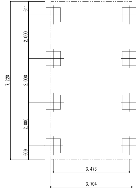
■ 基礎配置図
