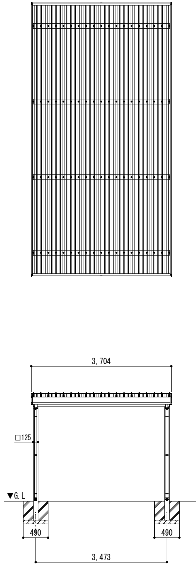
■ 接図
